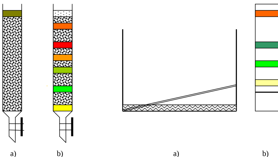
Obr. č. 1 Schéma uspořádání a průběhu (postupné eluce) kolonové (sloupcové) chromatografie
